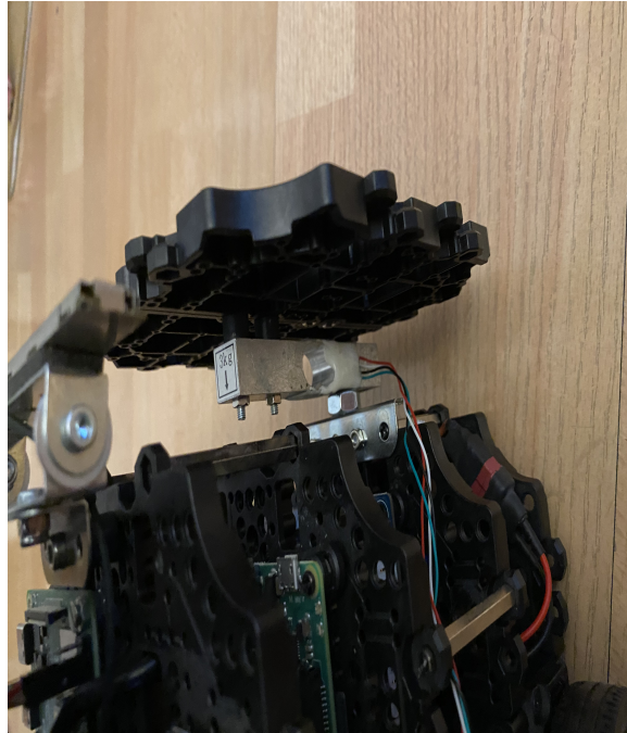
FIGURE 3.12 : Plaque permettant au robot de pousser les obstacles avec son capteur de force.
