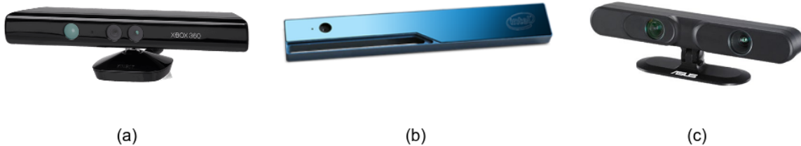
FIGURE 3.9 : Capteurs RGB et capteur de profondeur en un seul dispositif. (a) Kinect Xbox, intégrée à notre robot illustré à la Figure 3.4. (b) Intel RealSense (utilisée sur notre robot) intégrée à notre robot illustré à la Figure 3.5. Les performances de ce capteur en terme de qualité d'image et de rapidité dépassent les deux autres types illustrés ici. (c) Asus Xtion PRO, un autre capteur du même type d'une marque concourante, également très populaire en robotique.
