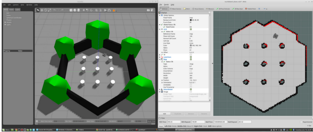
FIGURE 4.11 : Le robot à gauche de l'image évolue dans un environnement simulé il cartographie son environnement à l'aide d'un scanner laser et utilise l'optométrie des roues pour calculer son déplacement. À droite on voit le résultat de SLAM sous forme d'une carte avec la position des obstacles et la position du robot.
