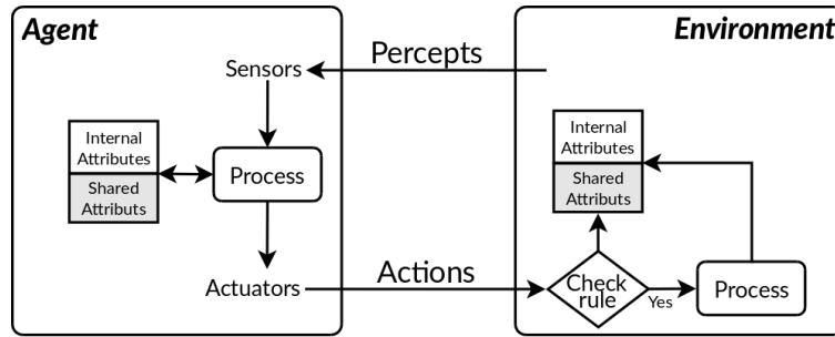
FIGURE 5.8 : Cette Figure illustre la relation entre un agent et son environnement. L'agent et l'environnement ont des attributs partagés et chacun d'eux a ses propres attributs qui le définissent. L'environnement est également composé de lois. Les agents agissent sur l'environnement par le biais d'actions. L'environnement peut directement modifier les attributs de l'agent si les lois sont transgressées.
