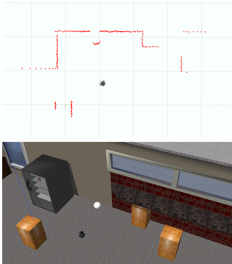
FIGURE 3.33 : En bas de l'image le robot Turtlebot 3 équipé d'un LIDAR dans un environnement domiciliaire simulé sous Gazebo. En haut, on voit, via RVIZ, le nuage de points généré par le LIDAR.
