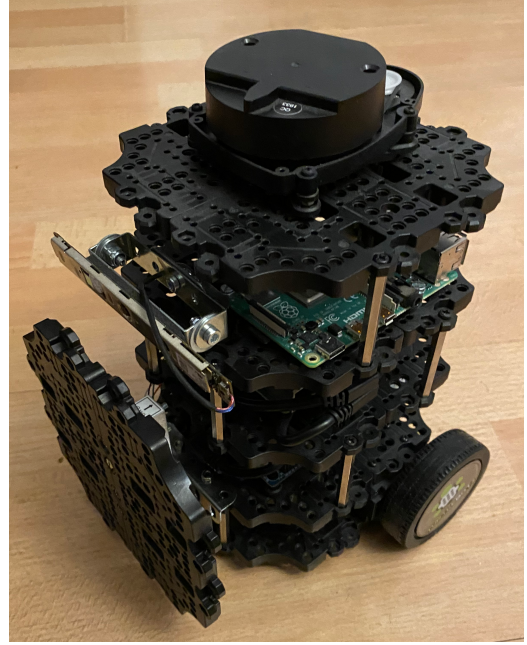
FIGURE 3.5 : Le robot Turtlebot 3 Burger sur lequel nous avons ajouté une caméra intel real sens SR300 et un capteur de force pour pousser les objets.
