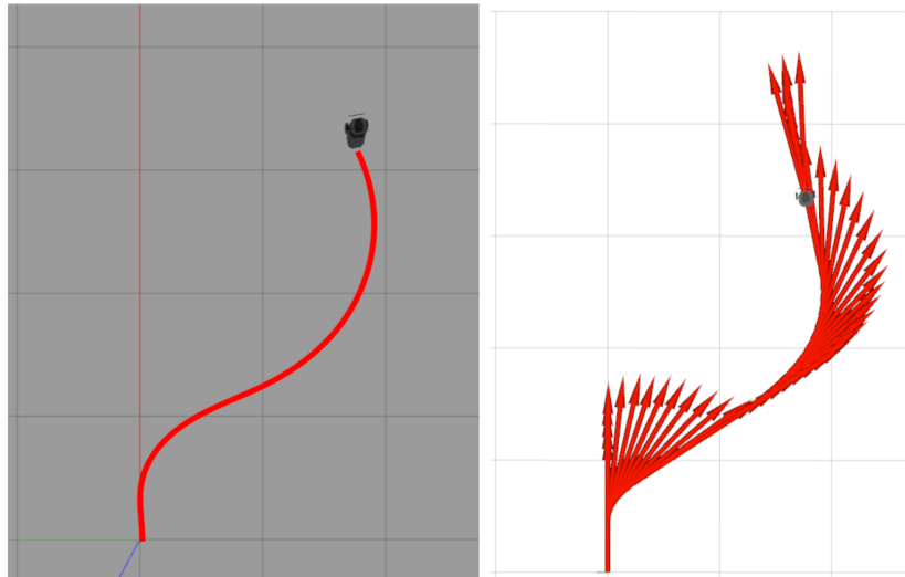
FIGURE 3.11 : À gauche la trajectoire du robot TurtleBot 3 sous le simulateur Gazebo , et à droite la visualisation sous RViz des vecteurs vitesse orientation des positions prises par le robot à chaque instant de son déplacement.
