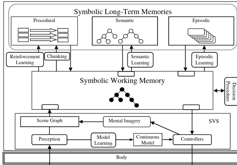
FIGURE 2.11 : Diagramme de l'architecture SOAR.
