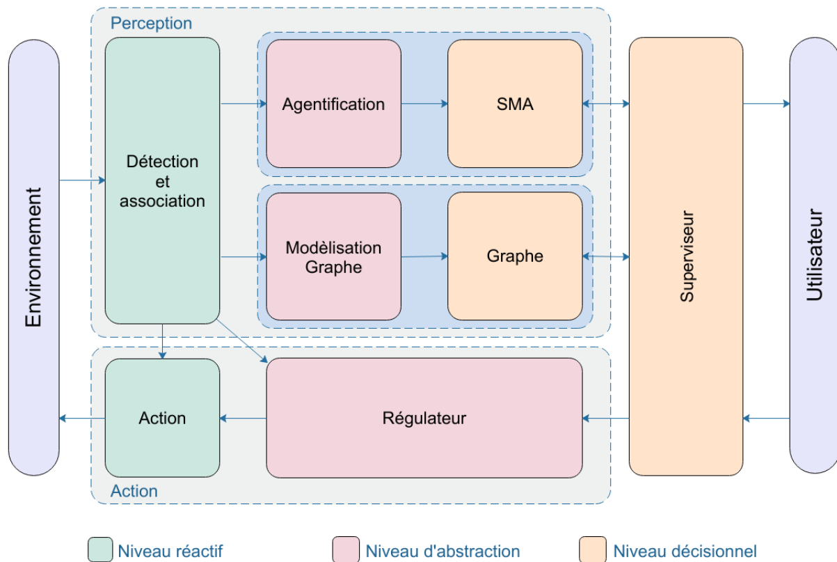
FIGURE 3.21 : Les principaux composants de l'architecture VICA : Le niveau cognitif regroupe le niveau d'abstraction et le niveau décisionnel.
