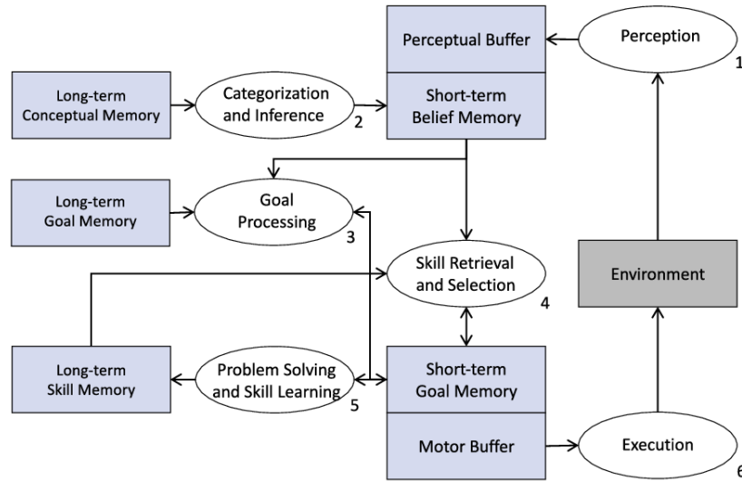
FIGURE 2.12 : Diagramme de l'architecture ICARUS, image extraite de [Choi and Langley, 2018]
