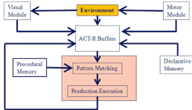
FIGURE 2.9 : Organisation des modules de ACT-R.
