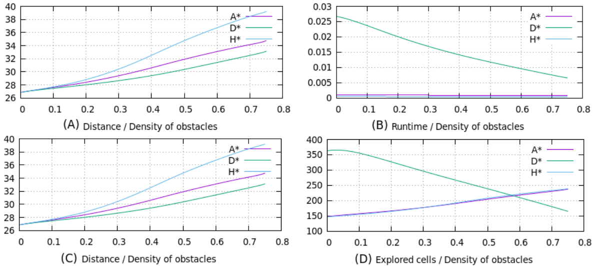
FIGURE 4.19 : Comparaison des distances, nombre de nœuds et temps d'exécution en seconde, entre les algorithmes H^* , D^* Lite et A^* .
