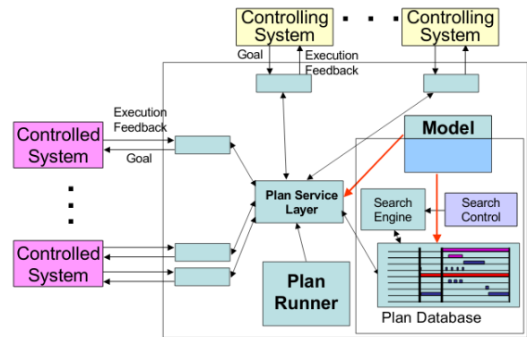
FIGURE 2.8 : Structure interne d'un agent IDEA. On trouve principalement trois sous-systèmes importants, le planificateur réactif, l'exécutif, et la base de plans.
