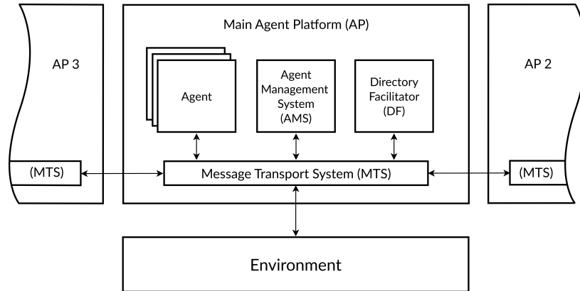
FIGURE 5.9 : Plateforme conforme FIPA à laquelle nous avons ajouté le module d’environnement ; la communication avec le module environnement et la plateforme s’effectue par échange de messages.
