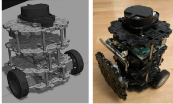
FIGURE 1.10 : Version du robot mobile utilisée plus récemment. Il s'agit d'une plateforme robotique commerciale connue sous le nom Turtlebot Burger .
