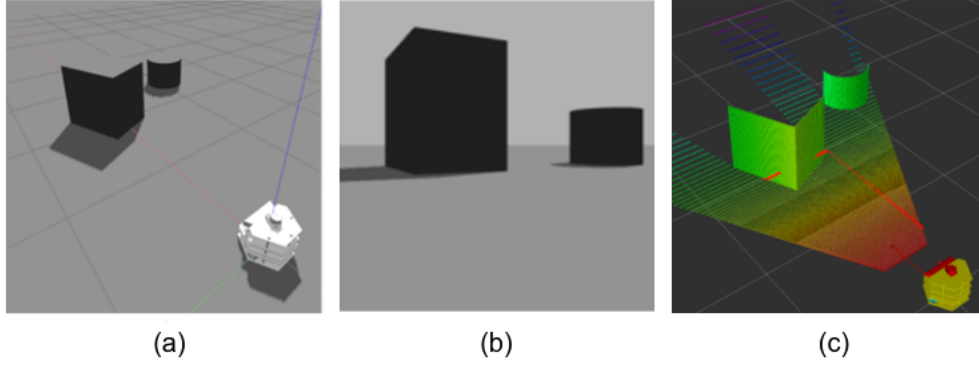
FIGURE 3.10 : Exemple du rendu en RGB et Nuage de point obtenu à l'aide du capteur Kinect. (a) Environnement du robot. (b) Camera RGB. (c) Nuage de point.
