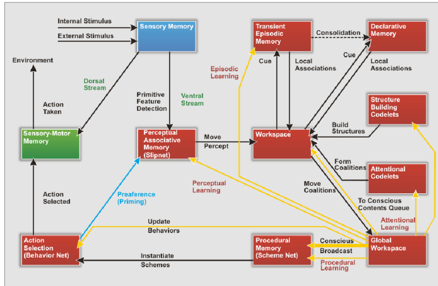
FIGURE 2.14 : Digramme de l'architecture LIDA.
