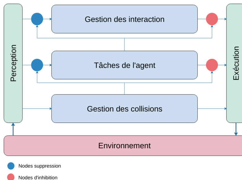
FIGURE 5.4 : Structure d'un agent réactif.
