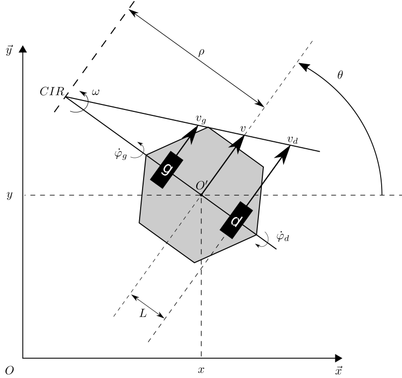
FIGURE 3.6 : Centre instantané de rotation
