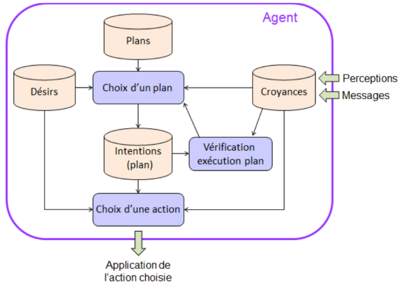
FIGURE 2.13 : Architecture interne d'un agent BDI. (Image extraite de [Taillandier et al., 2012])
