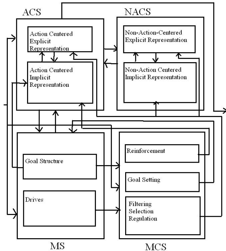
FIGURE 2.10 : Organisation de l'architecture CLARION.
