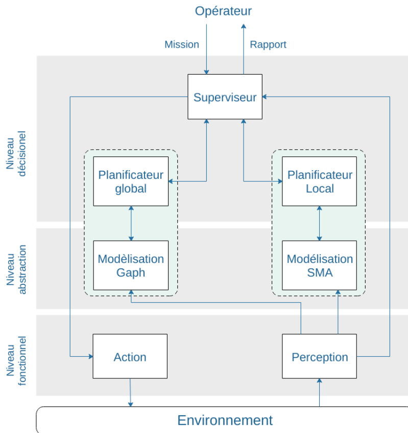
FIGURE 3.20 : Architecture VICA à trois niveaux.
