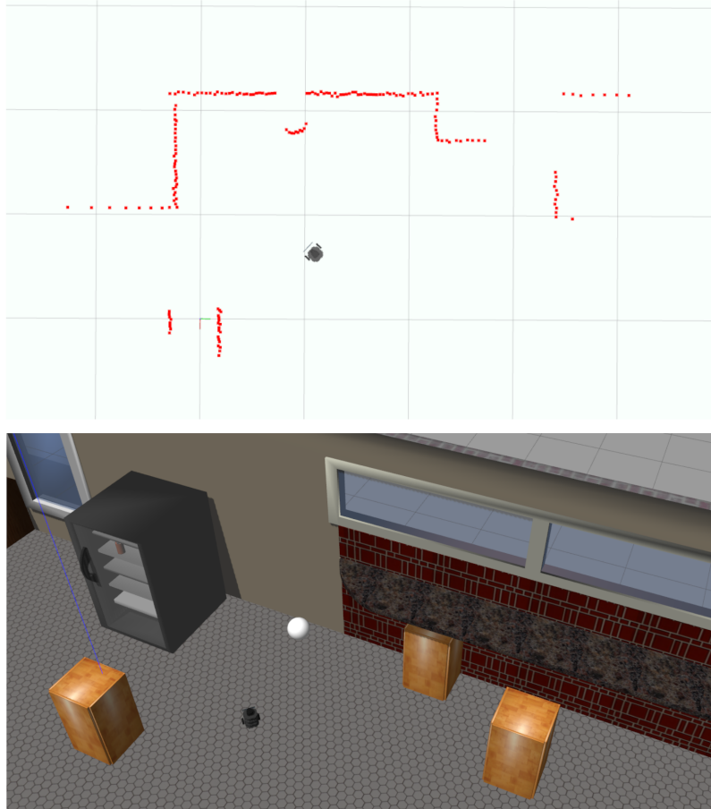
FIGURE 3.7 : En bas de l'image le robot Turtlebot 3 équipé d'un LIDAR dans un environnement domestique simulé sous Gazebo. En haut, on voit, via RVIZ, le nuage de points généré par le LIDAR.
