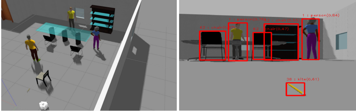
FIGURE 5.12 : Utilisation du système de reconnaissance dans Gazebo .
